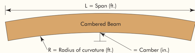
BEAM CAMBER PARAMETERS
